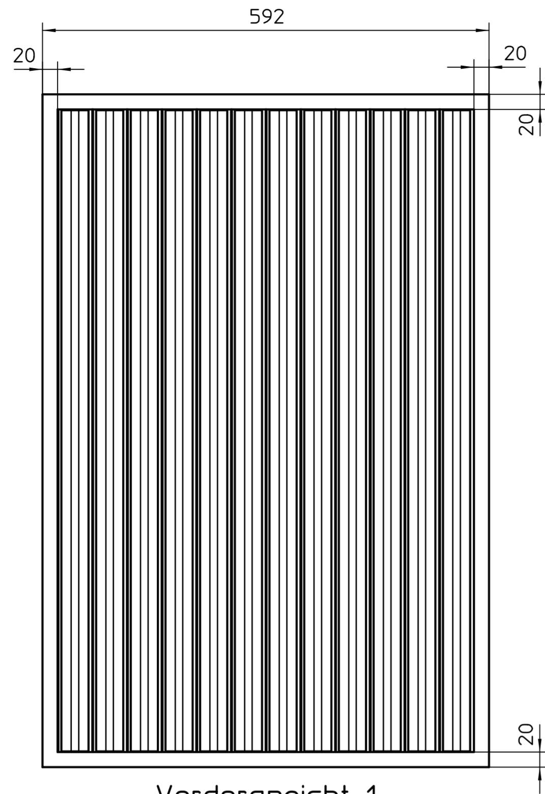
Vorderansicht 1
