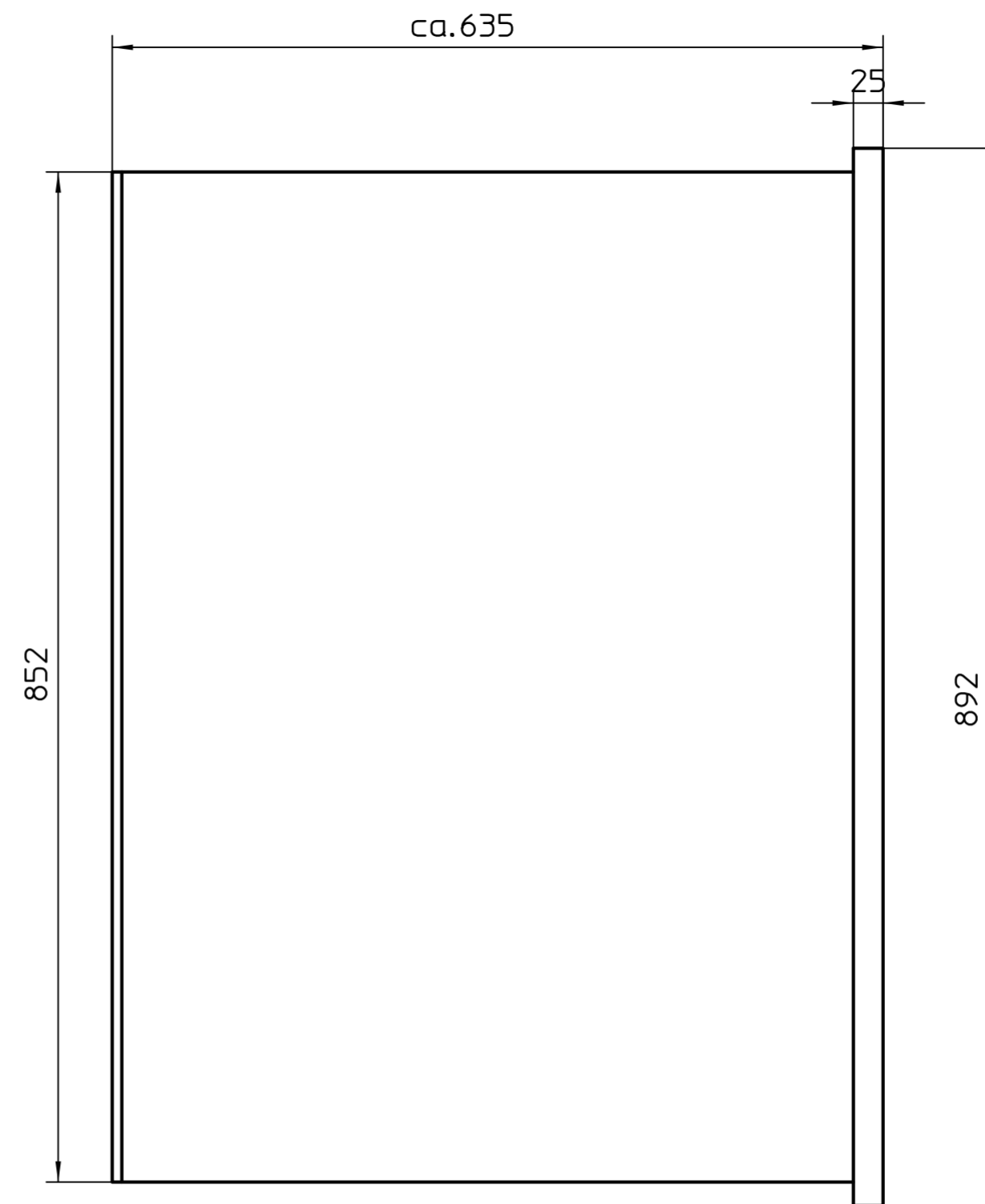
SA links 1
