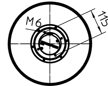
Rückansicht 1
