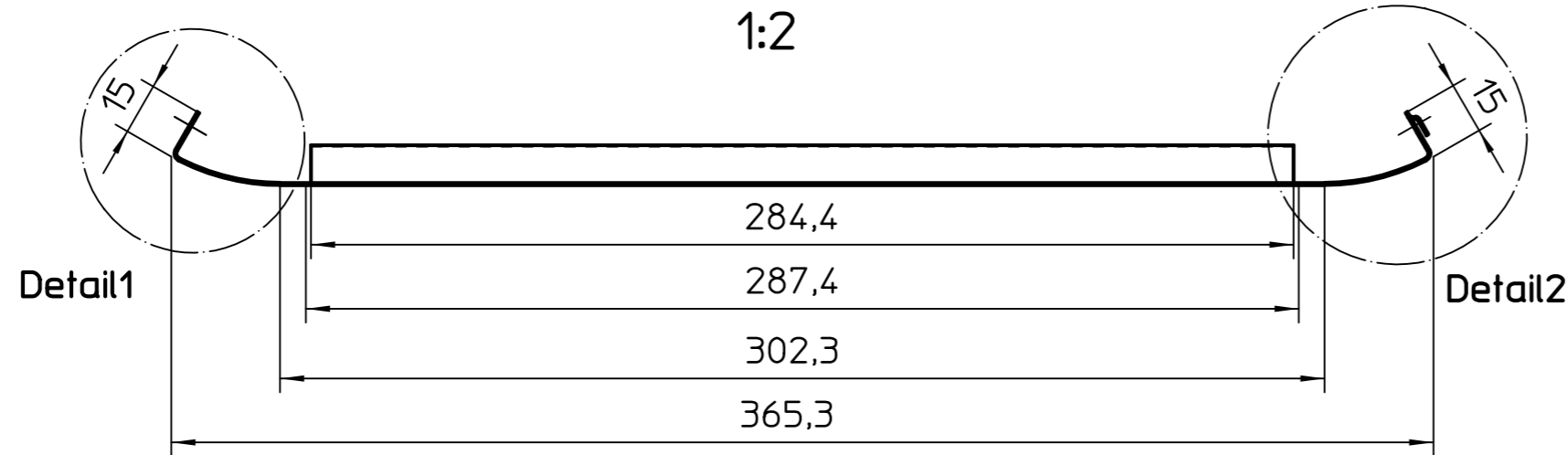
Draufsicht 1
