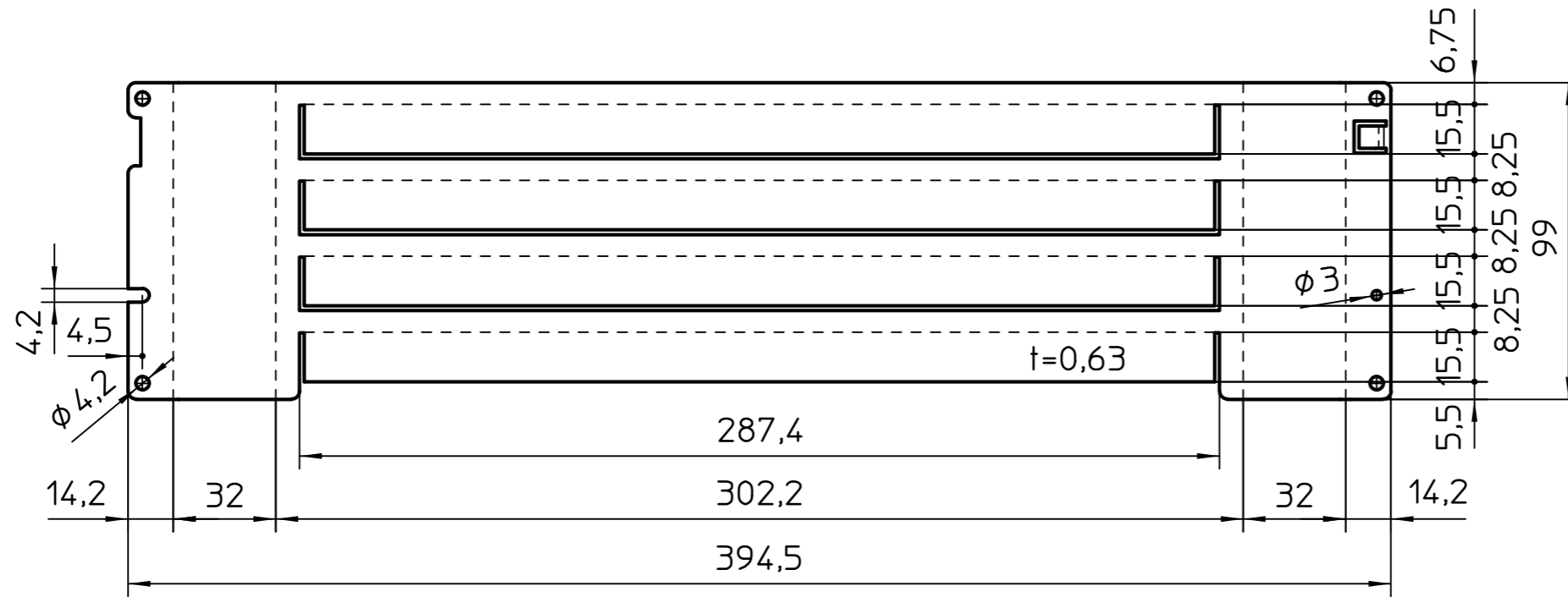
Abwicklung1
