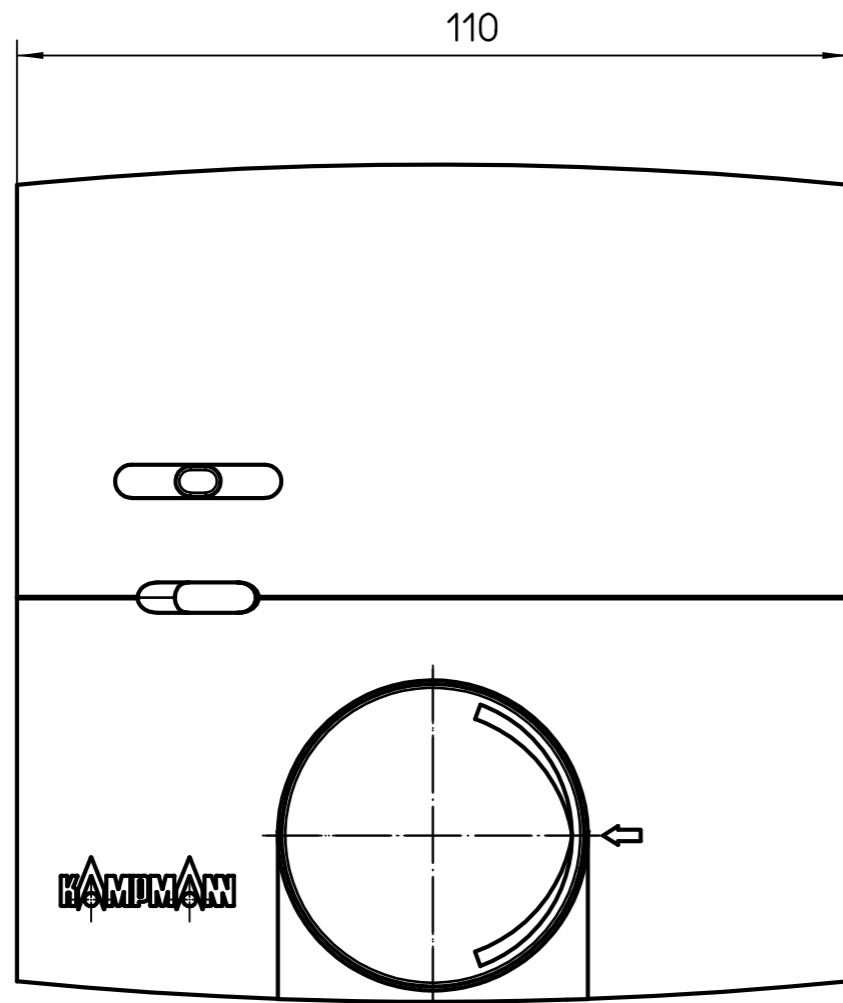
Vorderansicht1
