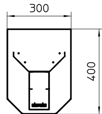
Draufsicht1
