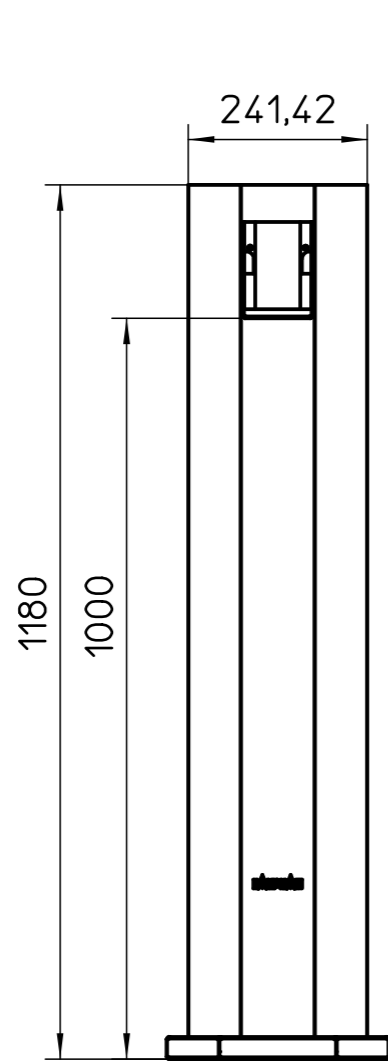
Vorderansicht1
